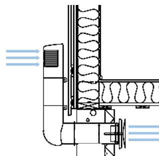
wentylacja dolnych kondygnacji budynku
